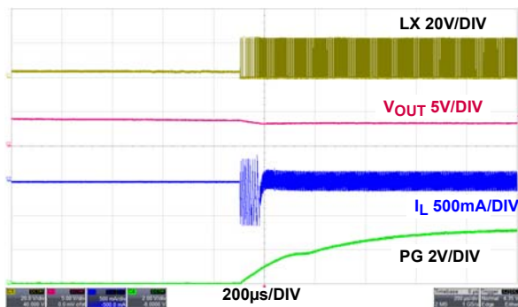
図 41. 逆電流保護動作からの回復、PWM
