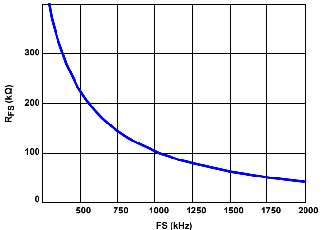
図 46. R_{FS} vs スイッチング周波数
