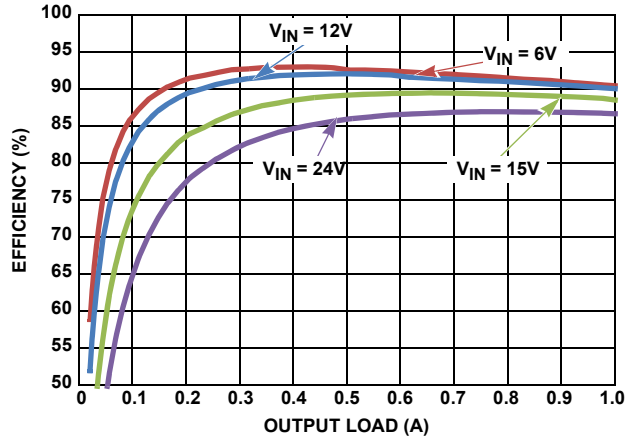
图 8. 效率 vs 負荷電流、PWM、 V_{OUT} = 5\text{V} , L1 = 30\mu\text{H}
