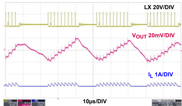
図 36. PFM モードから PWM モードへの切り替わり
