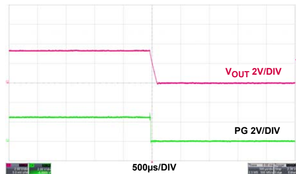
図 42. 過熱保護動作、PWM
