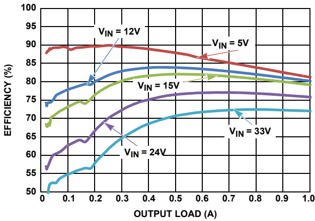
図 11. 効率 vs 負荷電流、PFM、 V_{OUT} = 1.8\text{V}
