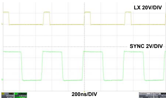
図 39. 1A 負荷時の同期信号、PWM
