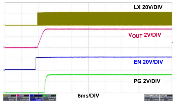
図 20. 無負荷時のスタートアップ、PWM
