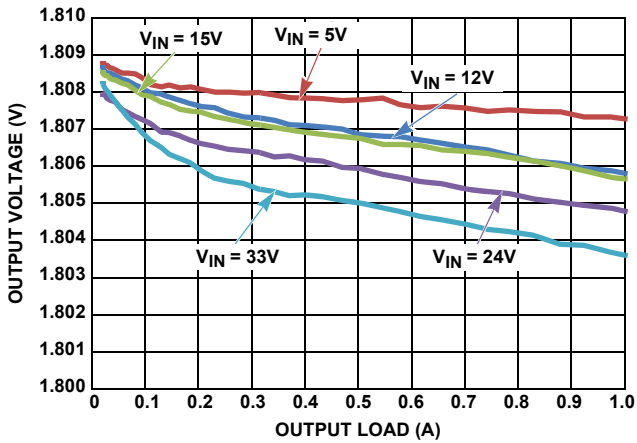
図 17. V_{OUT} レギュレーション vs 負荷電流、PWM、 V_{OUT} = 1.8\text{V}
