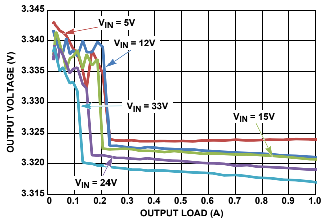
図 16. V_{OUT} レギュレーション vs 負荷電流、PFM、 V_{OUT} = 3.3\text{V}
