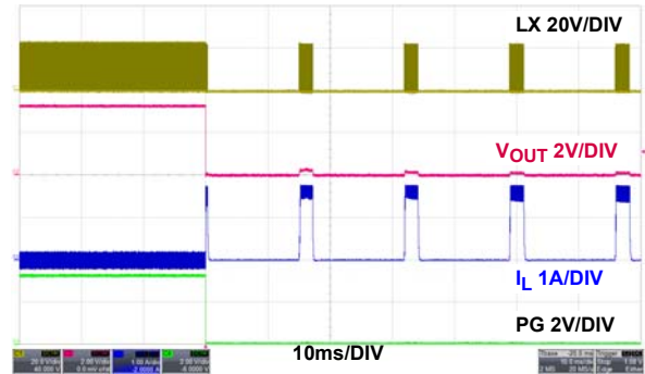
図 38. 過電流保護ヒューズモード動作、PWM
