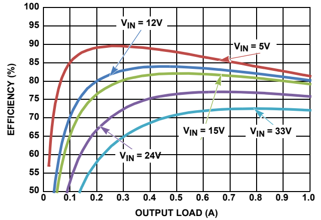
図 12. 効率 vs 負荷電流、PWM、 V_{OUT} = 1.8\text{V}
