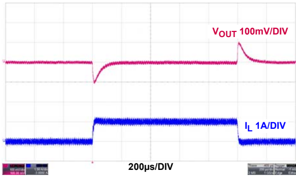
図 35. 負荷過渡応答、PWM
