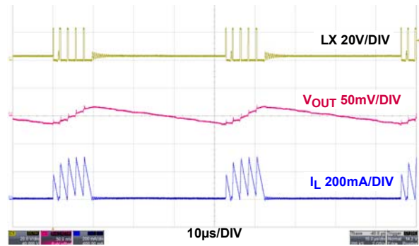
図 32. 20mA 軽負荷動作、PFM
