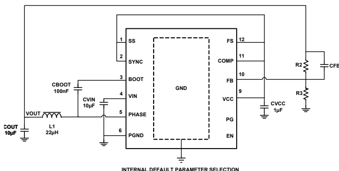
図 1. アプリケーション回路例
