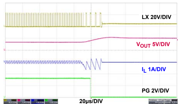
図 40. 逆電流保護動作、PWM
