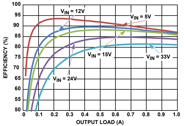
图 10. 效率 vs 負荷電流、PWM、 V_{OUT} = 3.3\text{V}
