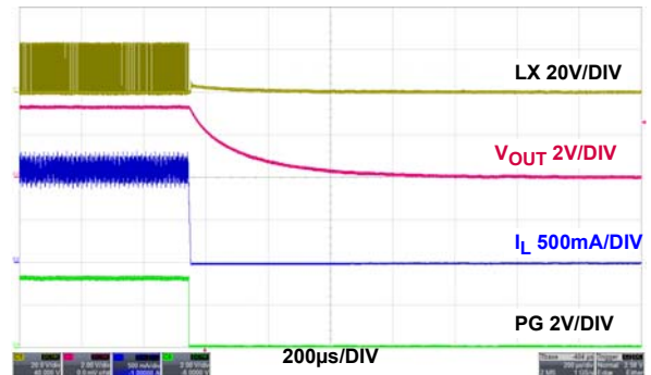
図 26. 1A 負荷時のシャットダウン、PFM
