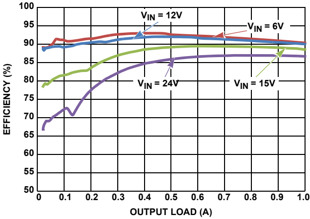
图 7. 效率 vs 負荷電流、PFM、 V_{OUT} = 5\text{V} , L1 = 30\mu\text{H}
