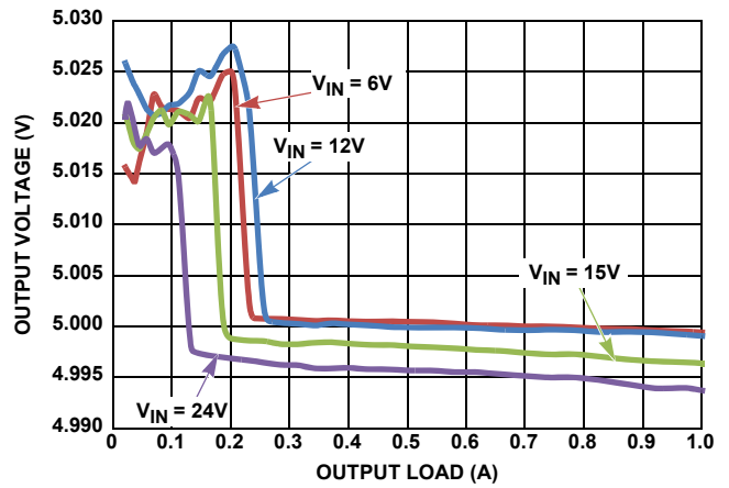
図 14. V_{OUT} レギュレーション vs 負荷電流、PFM、 V_{OUT} = 5\text{V} , L_1 = 30\mu\text{H}
