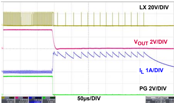
図 37. 過電流保護動作、PWM
