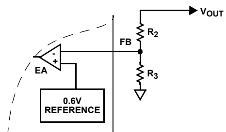
図 45. 外付け抵抗分圧回路
