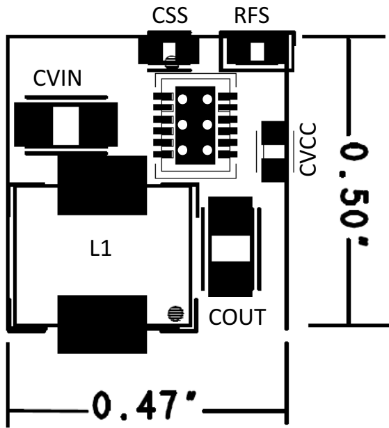
図 50. プリント基板の電源層とアイランド
