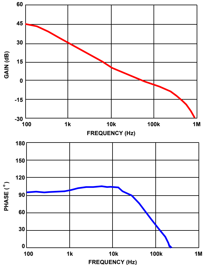
図 49. ループゲインのシミュレーション結果
