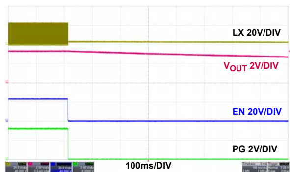
図 22. 無負荷時のシャットダウン、PWM
