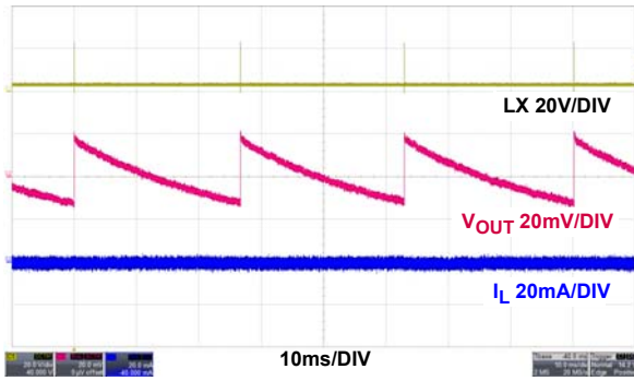
図 29. 無負荷時の定常状態動作、PFM
