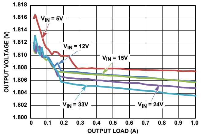
図 18. V_{OUT} レギュレーション vs 負荷電流、PFM、 V_{OUT} = 1.8\text{V}
