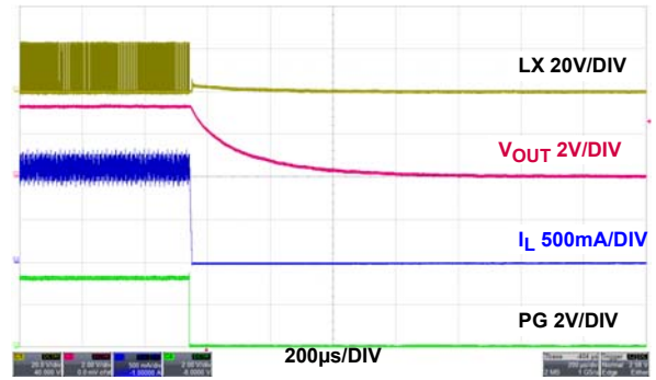
図 24. 1A 負荷時のシャットダウン、PWM
