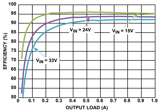
图 6. 效率 vs 負荷電流、PWM、 V_{OUT} = 12\text{V}
