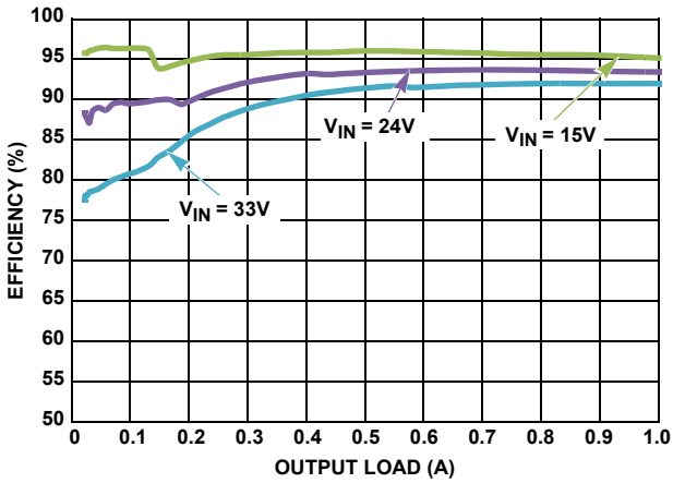
图 5. 效率 vs 負荷電流、PFM、 V_{OUT} = 12\text{V}
