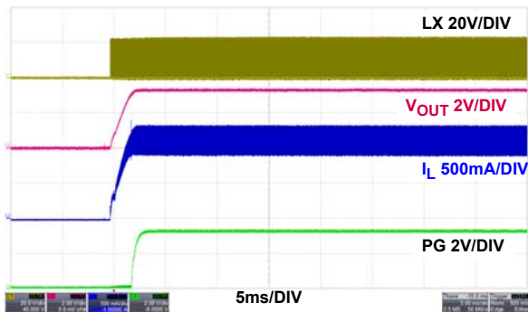
図 25. 1A 負荷時のスタートアップ、PFM
