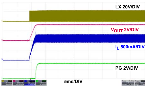
図 23. 1A 負荷時のスタートアップ、PWM
