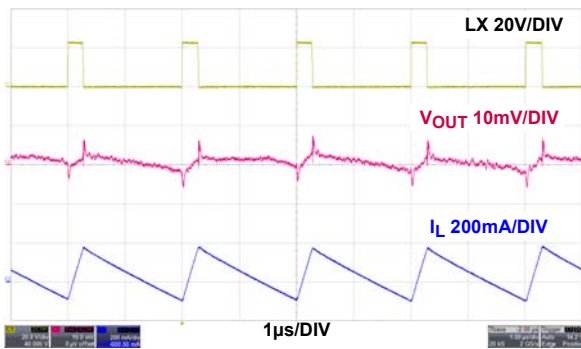
図 33. 20mA 軽負荷動作、PWM
