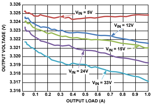
図 15. V_{OUT} レギュレーション vs 負荷電流、PWM、 V_{OUT} = 3.3\text{V}
