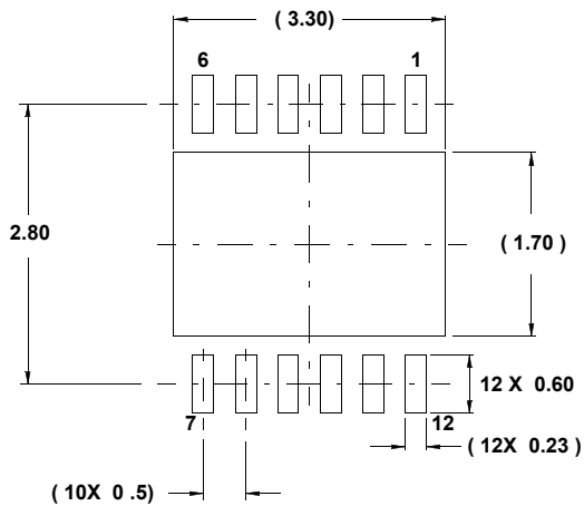
推奨ランドパターンの例
