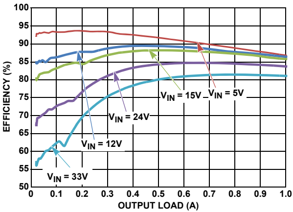
图 9. 效率 vs 負荷電流、PFM、 V_{OUT} = 3.3\text{V}
