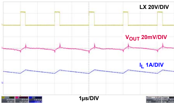
図 31. 1A 負荷時の定常状態動作、PWM
