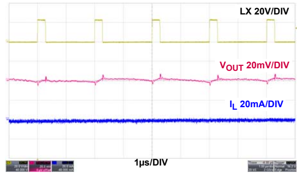
図 30. 無負荷時の定常状態動作、PWM
