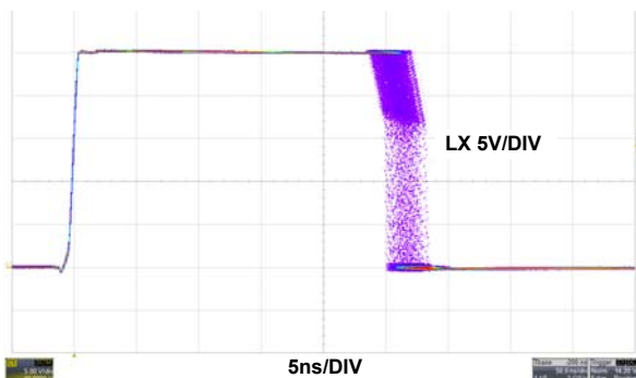
図 27. 無負荷時のジッタ、PWM
