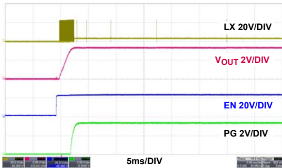
図 19. 無負荷時のスタートアップ、PFM
