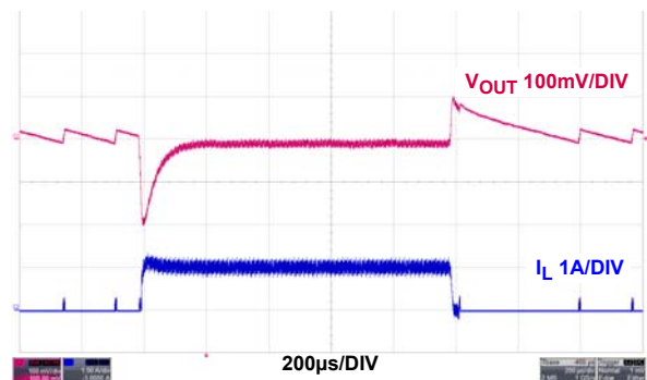
図 34. 負荷過渡応答、PFM
