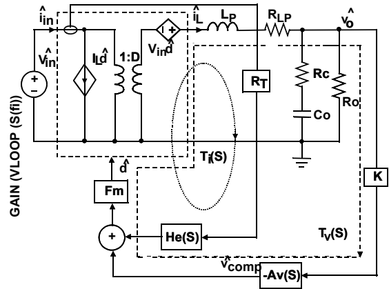
図 47. 同期整流型降圧レギュレータの小信号モデル
