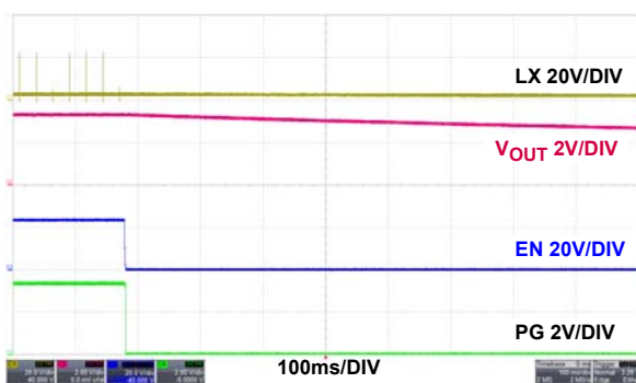
図 21. 無負荷時のシャットダウン、PFM
