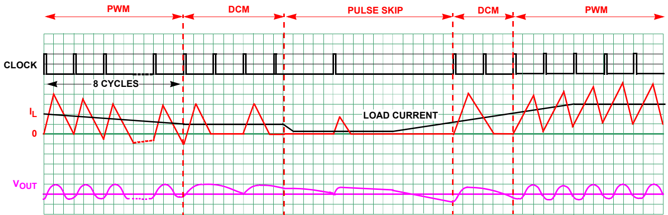
図 43. 電流不連続モード動作波形
