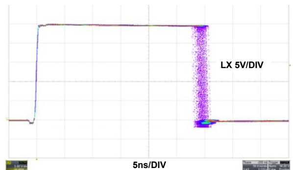
図 28. 1A 負荷時のジッタ、PWM
