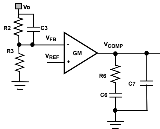
図 48. タイプ II 補償回路
