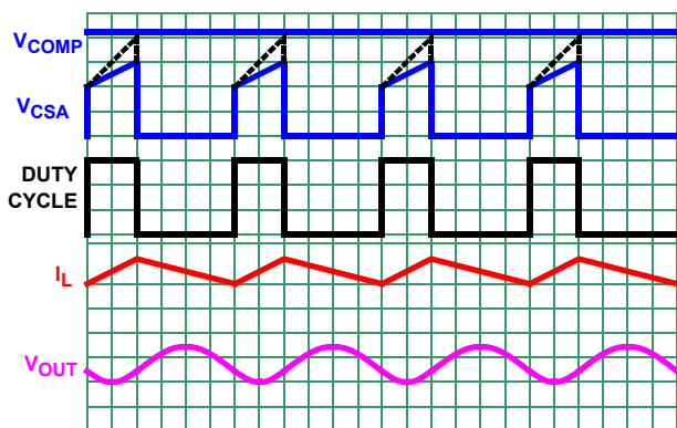
図 44. PWM 動作波形
